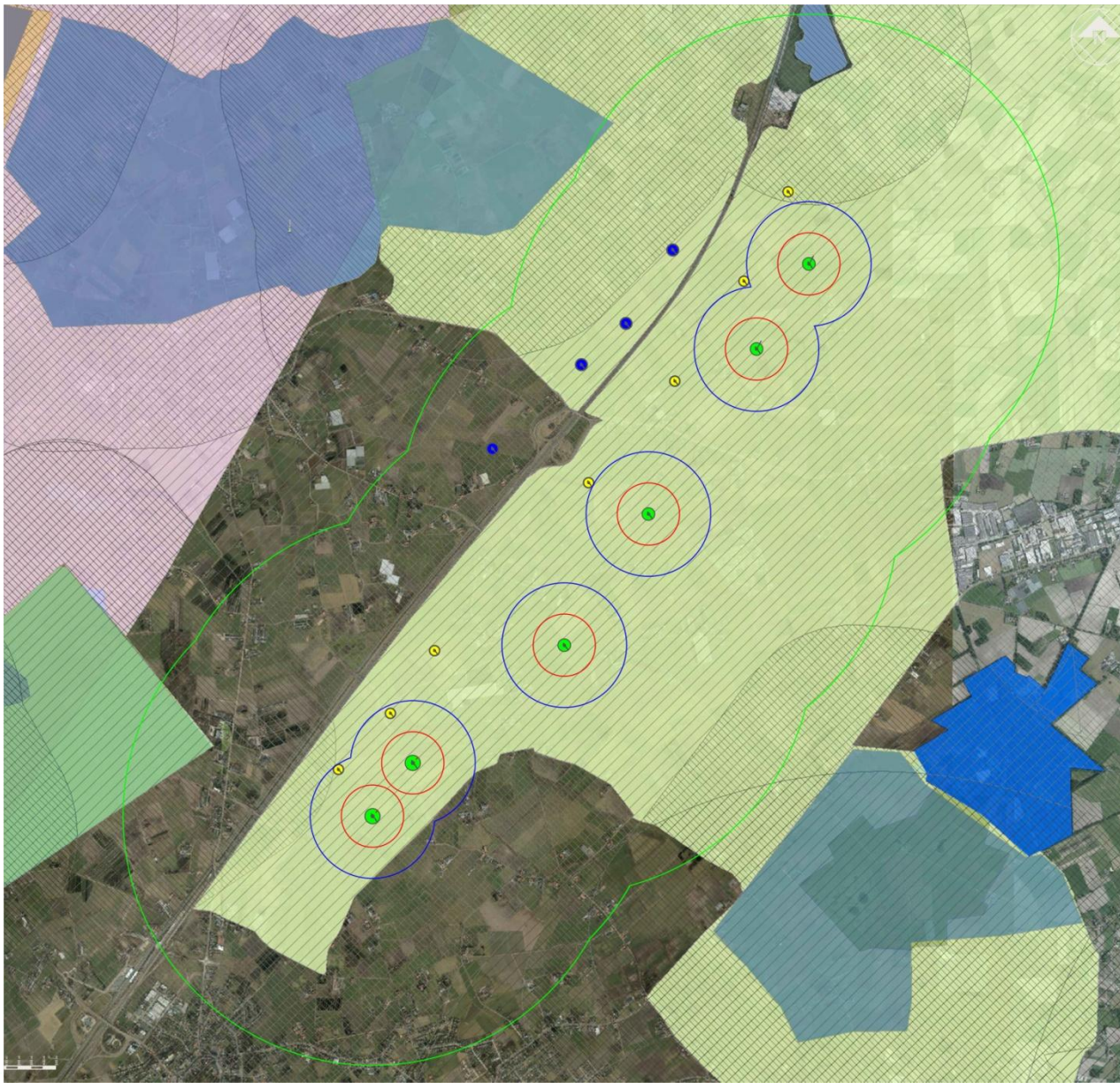
Project Hoogstraten - Plaatsing van zes bijkomende windturbines. Weergave van de risicozones voor Avifauna.
